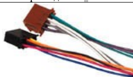
Kabli za avto radio ISO-konektori
